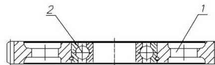
Рис.4 КР-2,4.01.400.00 – Колесо зубчатое
